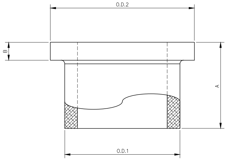
FLANGE ADAPTER SCALE: NTS
