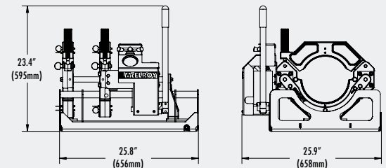
DYNAMC 28 HP 2-JAW
