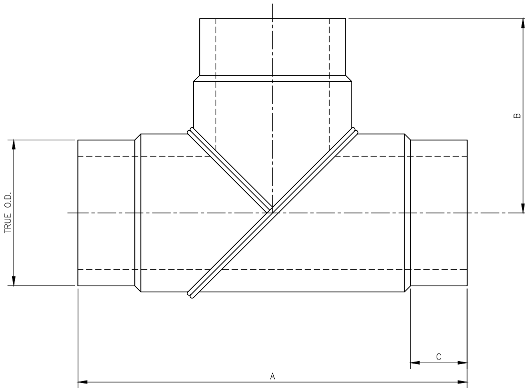
EQUAL TEE SCALE: 1"=1'-0"
