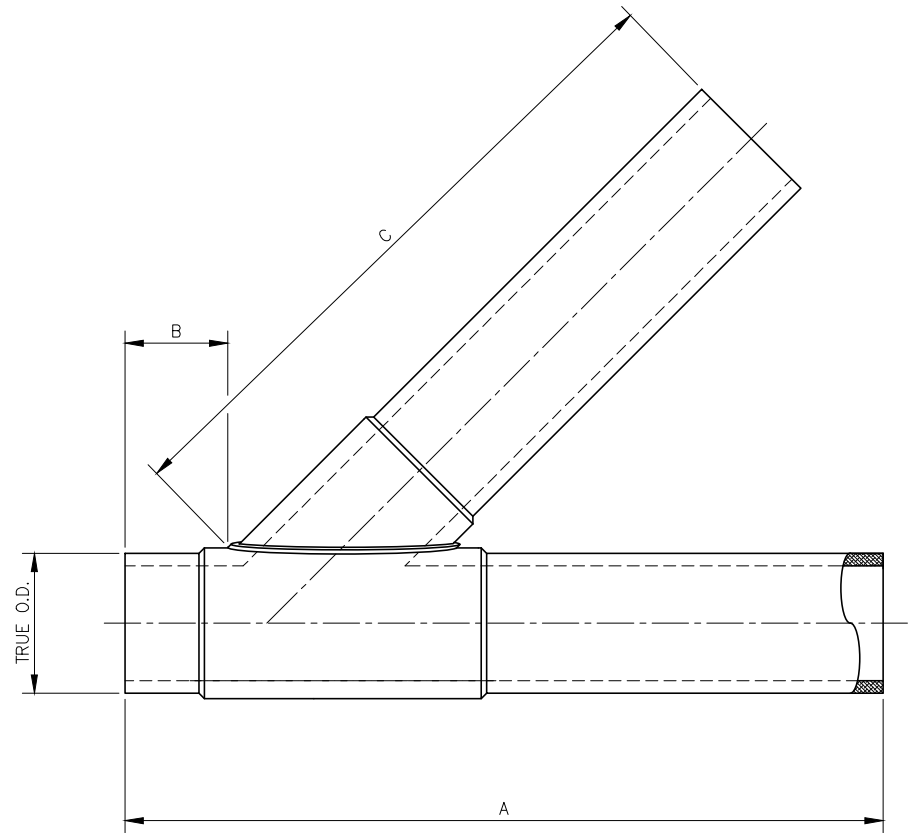
LATERAL WYE SCALE: NTS
